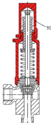
Figur 963 gastät kåpa
