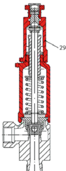
Figur 962 öppet lättverk
