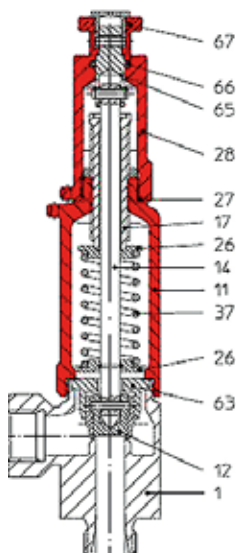
Figur 961 slutet lättverk
